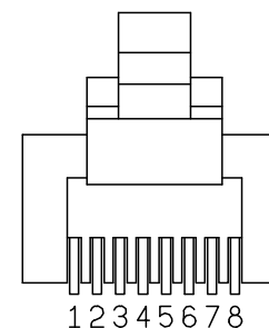
RJ45-8pins_連接側圖位
