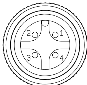
M12-4pins(公)_外牙_連接側圖位
