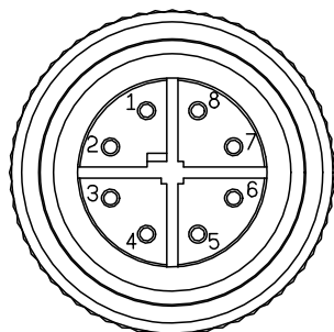
M12-8pins(公) 連接側腳位
